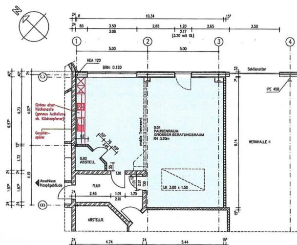
Grundriss Küche/Konferenzraum
