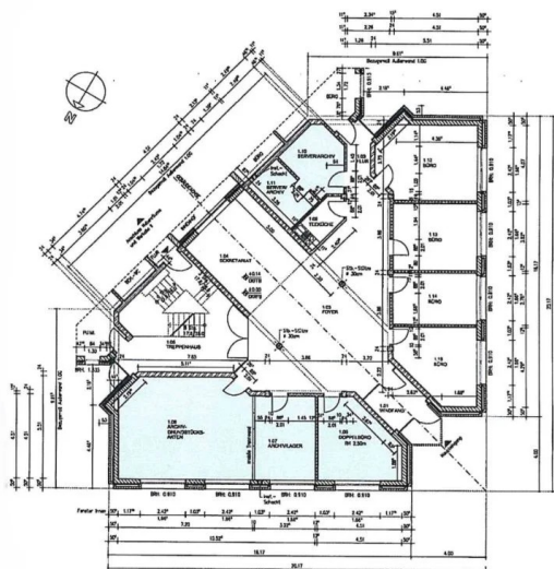
Grundriss
