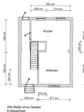
Grundriss Erdgeschoss
