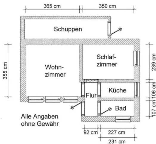
Grundriss
