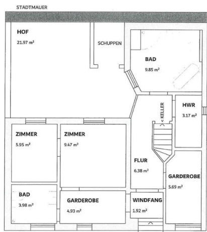
Grundriss Erdgeschoss
