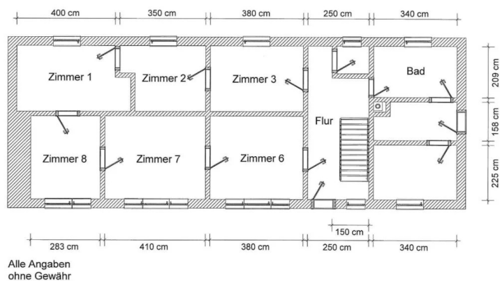
Grundriss
