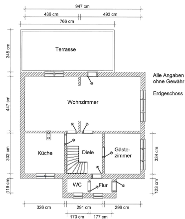
Grundriss Erdgeschoss
