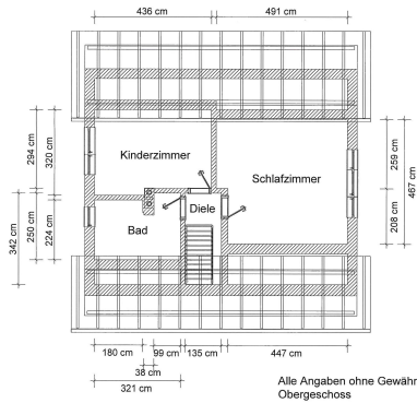
Grundriss Obergeschoss
