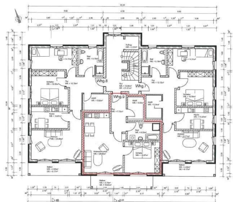
Grundriss
