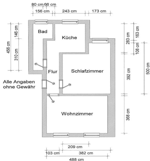
Grundriss
