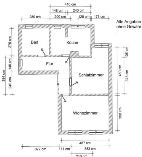
Grundriss
