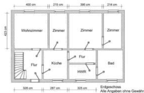
Grundriss Erdgeschoss
