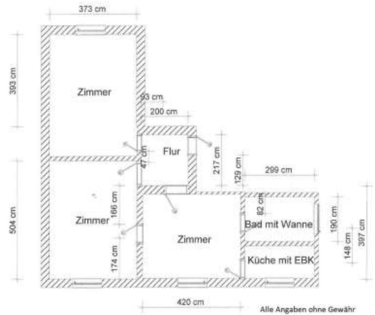
Grundriss
