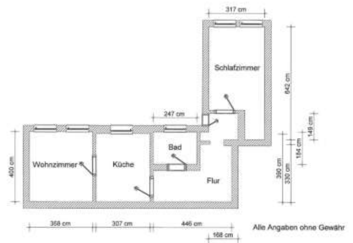
Grundriss
