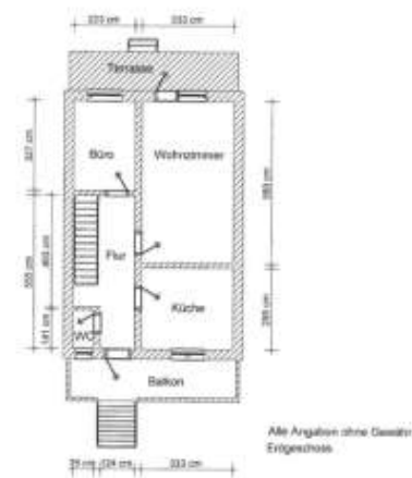
Grundriss Erdgeschoss
