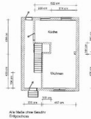
Grundriss Erdgeschoss
