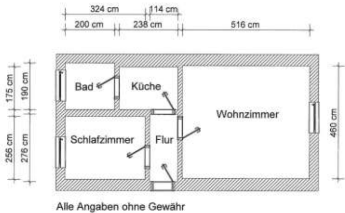
Grundriss
