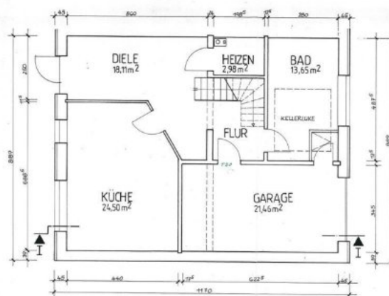
Grundriss Erdgeschoss
