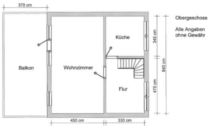
Grundriss OG
