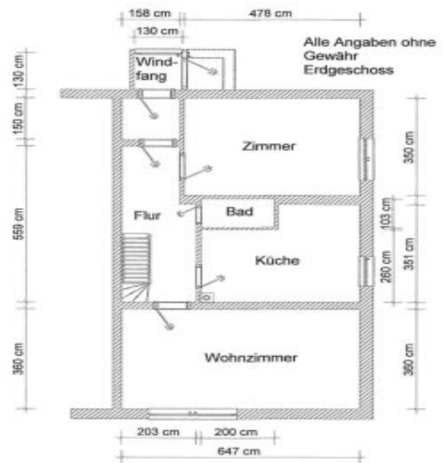
Grundriss Erdgeschoss
