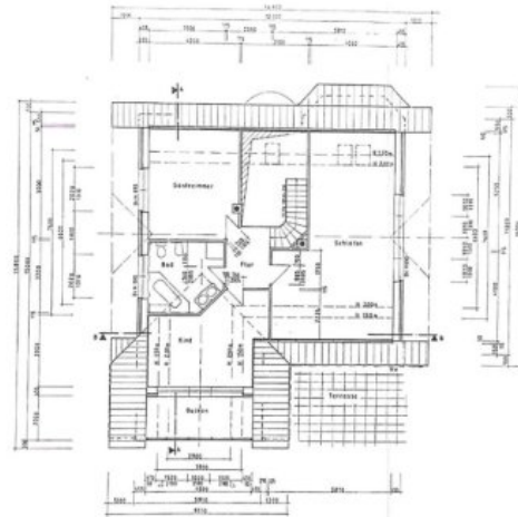
Grundriss Obergeschoss
