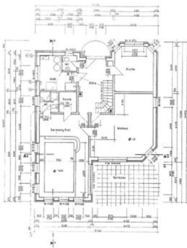
Grundriss Erdgeschoss
