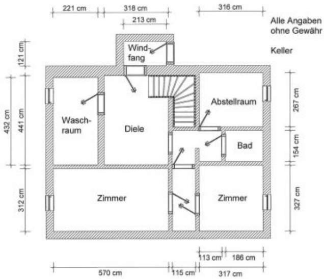
Grundriss Keller
