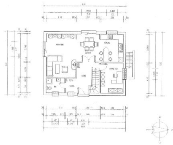
Grundriss Erdgeschoss
