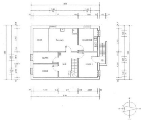
Grundriss Keller
