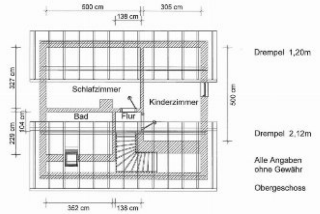
Grundriss Obergeschoss
