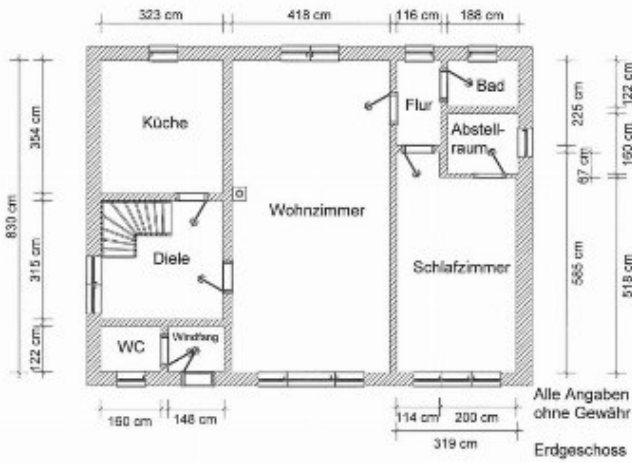
Grundriss Erdgeschoss
