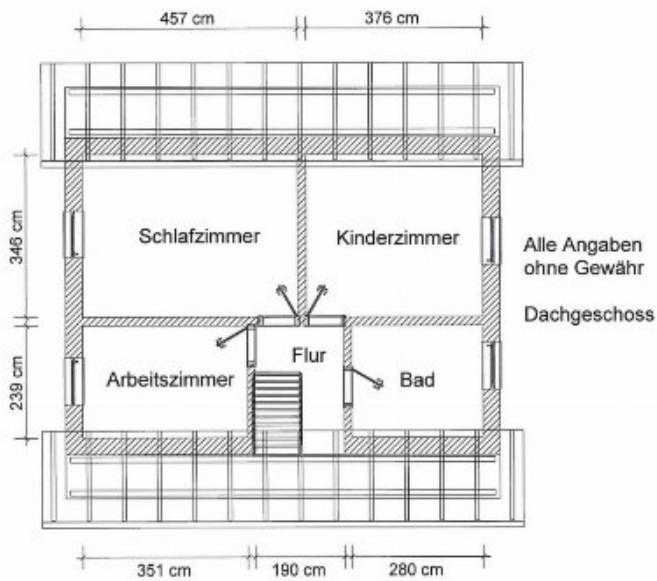
Grundriss Obergeschoss
