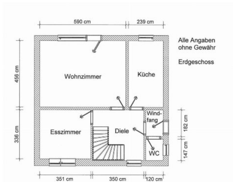
Grundriss Erdgeschoss
