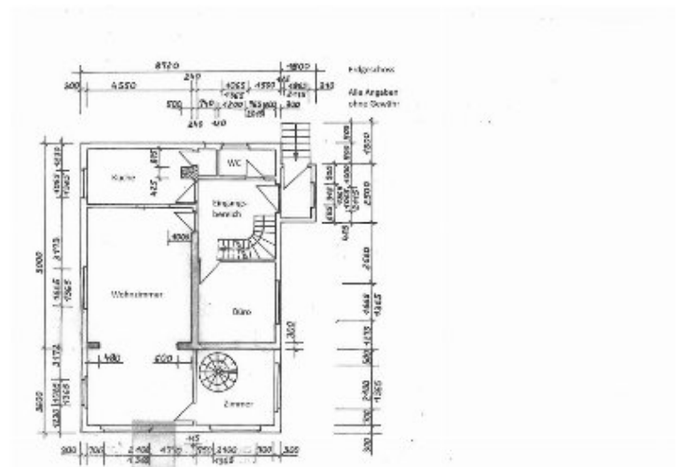
Grundriss Erdgeschoss
