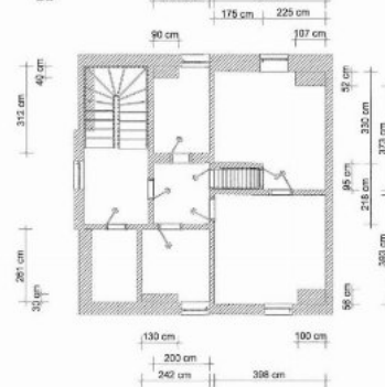
Grundriss Dachgeschoss
