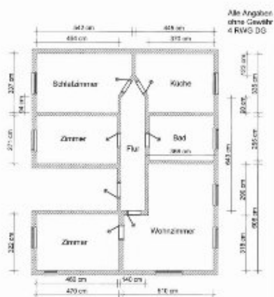
Grundriss
