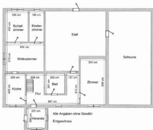
Grundriss Erdgeschoss
