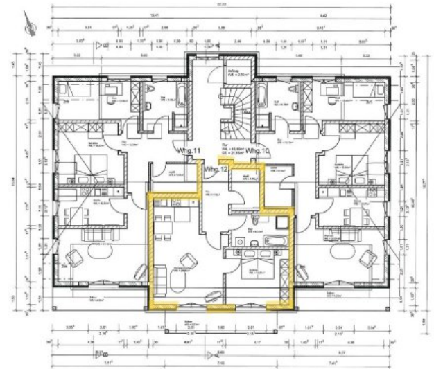
Grundriss
