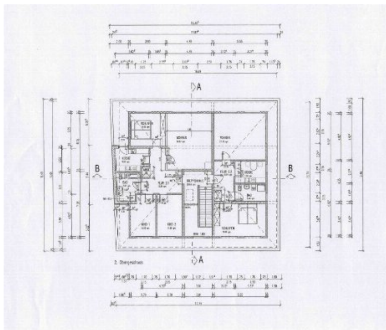
Grundriss 2. Obergeschoss
