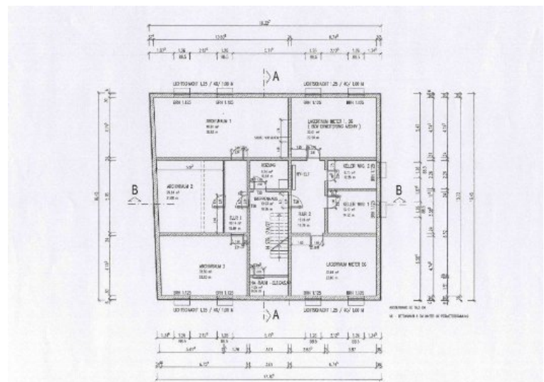
Grundriss Kellergeschoss
