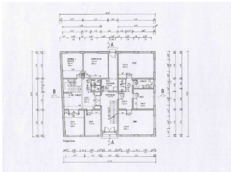
Grundriss Erdgeschoss
