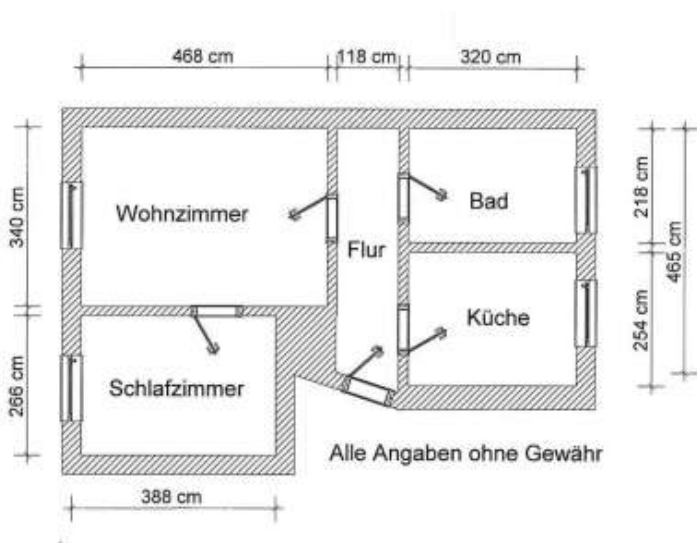
Grundriss
