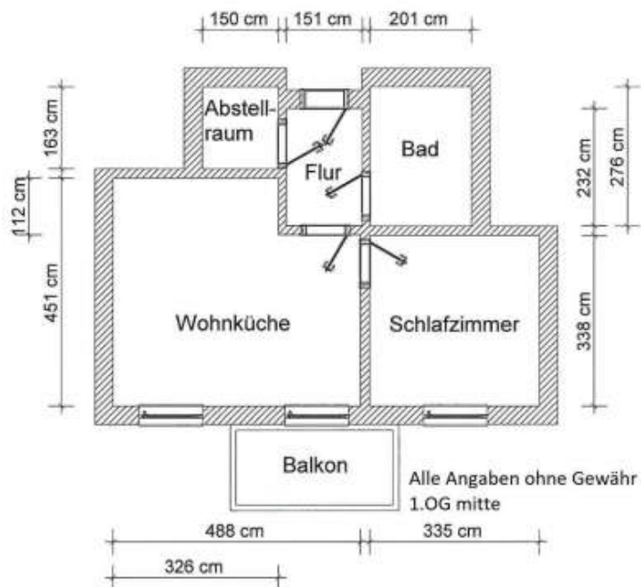
Grundriss
