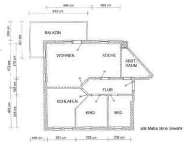
Grundriss
