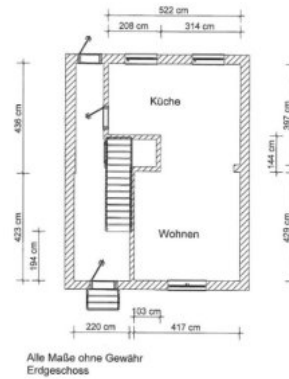
Grundriss Erdgeschoss
